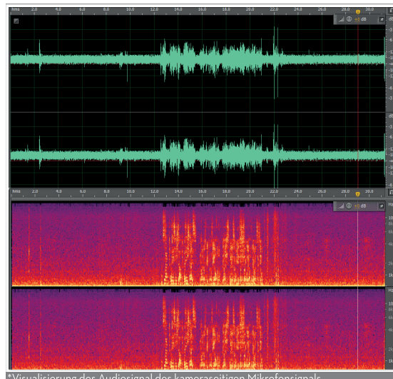
*Visualisierung des Audiosignal des kameraseitigen Mikrofonsignals
