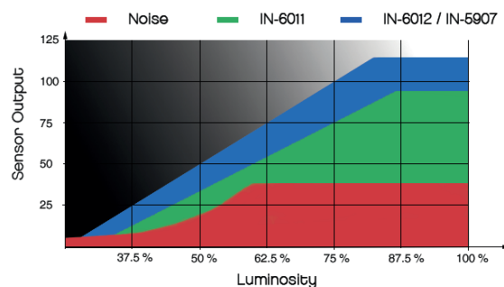
Abb. Der erweiterte Dynamikbereich von 94 dBi der IN-6011 HD mit der hohen Sensorempfindlichkeit und außergewöhnlichen Signal-zu-Rauschen Verhältnis wird nur von unserer WDR Line überboten.
